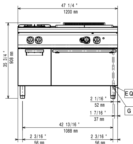
Oldalnézet
